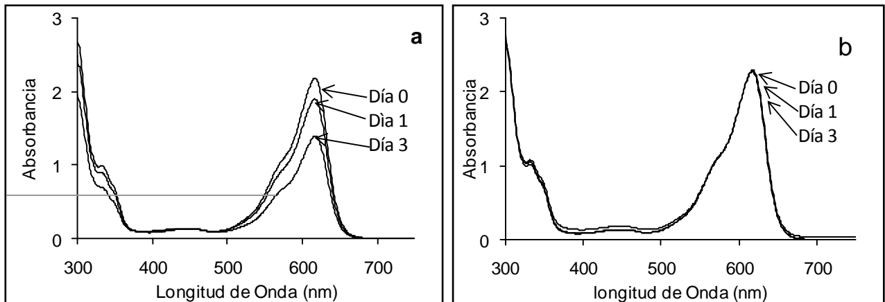
Figura 2. Espectro UV-Vis en de IA (6,99 x 10 -4 M) en solución HMPA vs. tiempo. a) Expuesta a la luz solar directa, a 28 ± 1 °C. b) En ausencia de luz.
