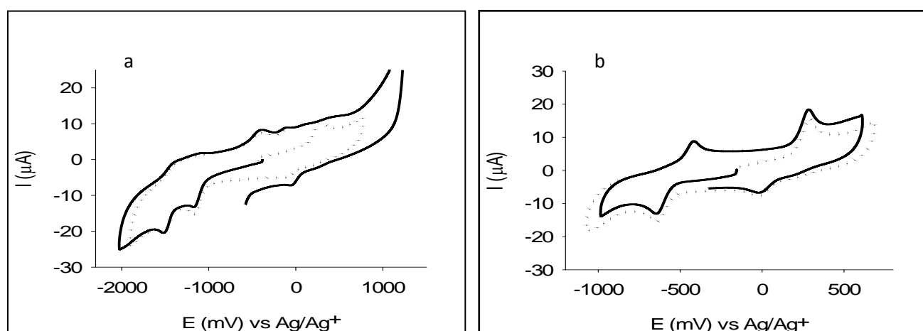
Figura 4. Comportamiento VC de 0,35mM IA en solución de DMF seco y desaireado; vb: 200 mV/s; ET: Carbono vítreo; CE: Chapa de Platino; ER: Ag/Ag + ; ES: 0,1M NaClO 4 en DMF, para barrido anódico (.....) y catódico (—) en a ) ausencia de TFA, b ) en presencia de 10 mM TFA.
