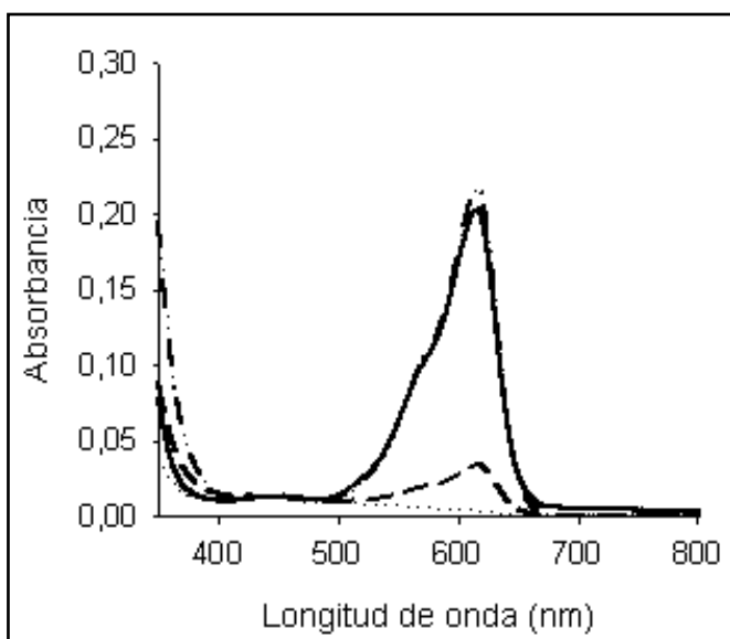
Figura 2. Espectro UV-Vis en de IA (6,99 x 10 -4 M) en solución HMPA vs. tiempo. a) Expuesta a la luz solar directa, a 28 ± 1 °C. b) En ausencia de luz.
