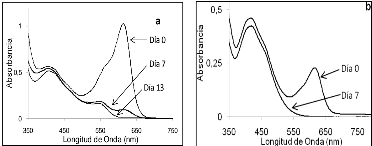
Figura 1. Espectro UV-Vis en función del tiempo de exposición a la luz de: a) IA (5,09 x 10 -4 M) en TMU; b) IA (5,72 x 10 -4 M) en NMP.
